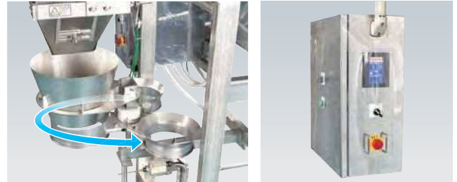
● 回転式切替受けシュート
