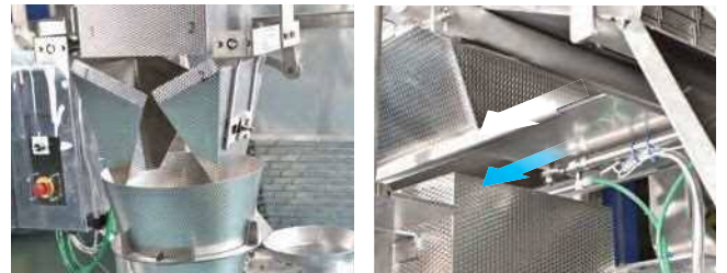
● 開閉ホッパー
